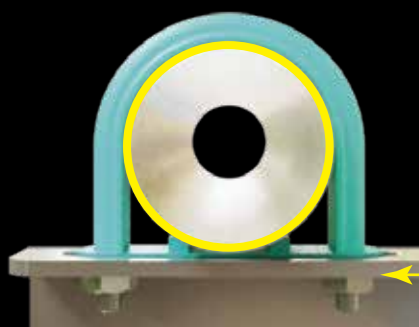
3. Uボルトをかぶせ、ナットを仮付する
