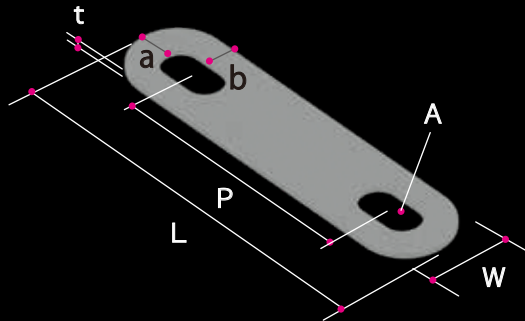
フッ素樹脂プレート
