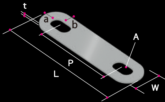
ポリプロピレン樹脂プレート
