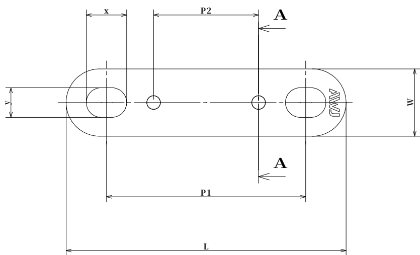
断面 A-A
